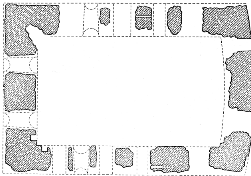
7. PLAN AV KÄLLARVÅNINGEN.
