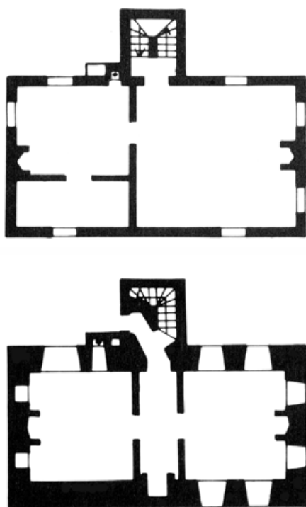
Sven Rosborns rekonstruktion av Kompanihuset i Malmös planlösning.
